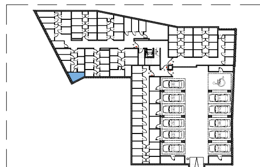
PIWNICA
